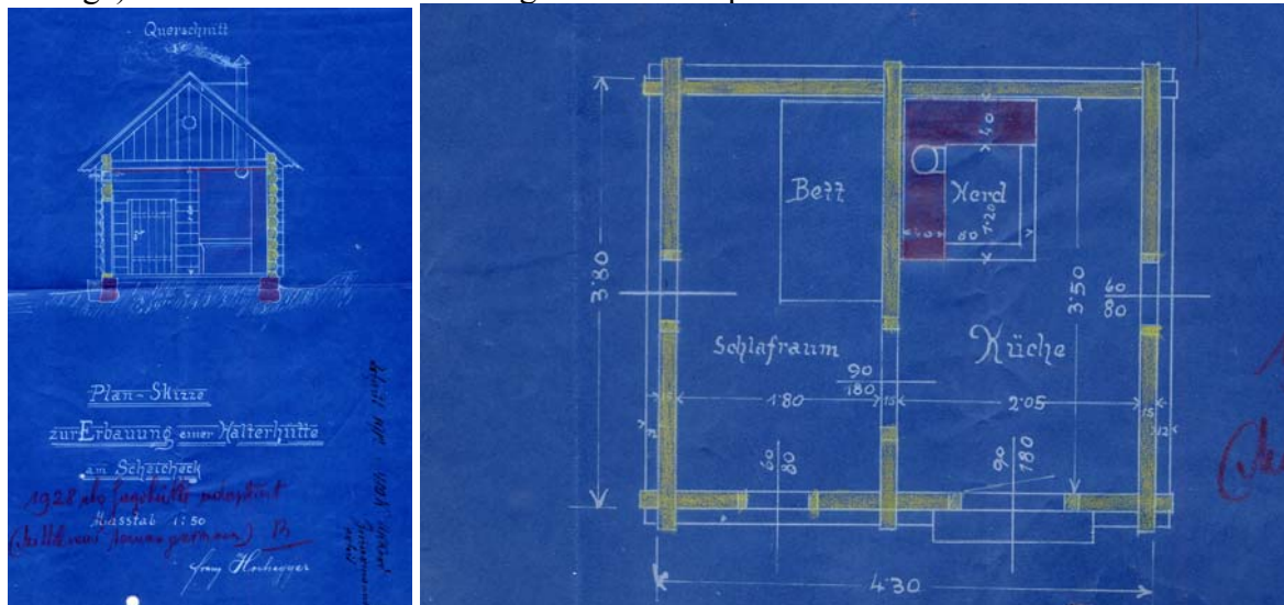
Stmk. LF., Aufriss und Grundriss der Halterhütte auf der Scheueckalm 1912.
